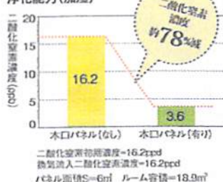
「杉木口スリット材」による二酸化窒素浄化能力(加湿)
