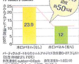
「杉木口スリット材」によるホルムアルデヒド浄化能力(加湿)
