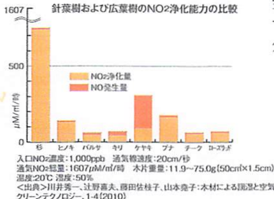
針葉樹および広葉樹のNO 2 浄化能力の比較
